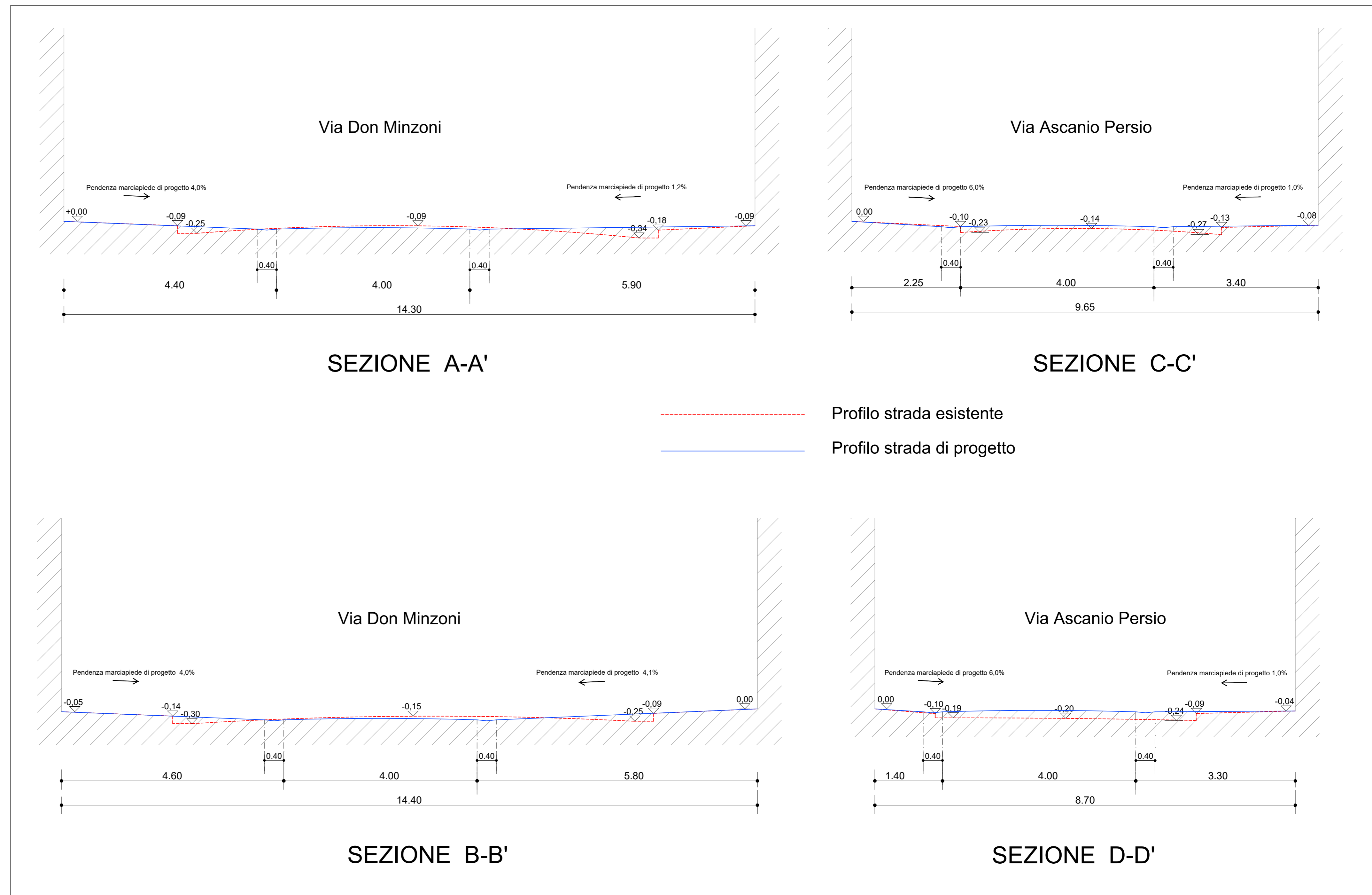
SEZIONI scala 1:100
